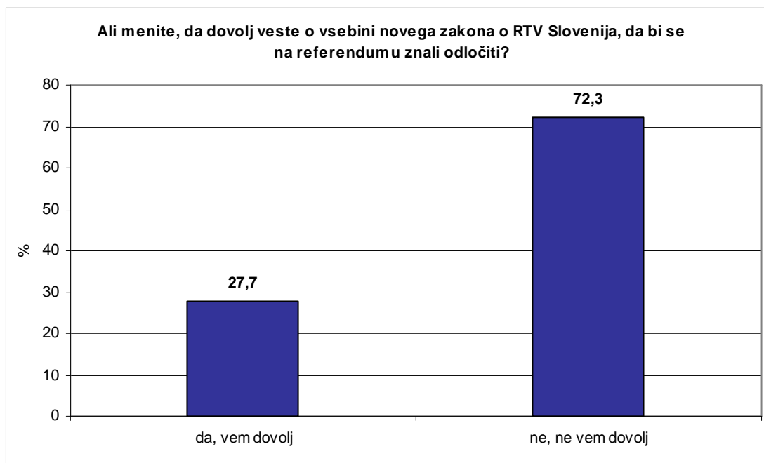
Slika 9. Informiranost o vsebini novega zakona o RTV Slovenija.
