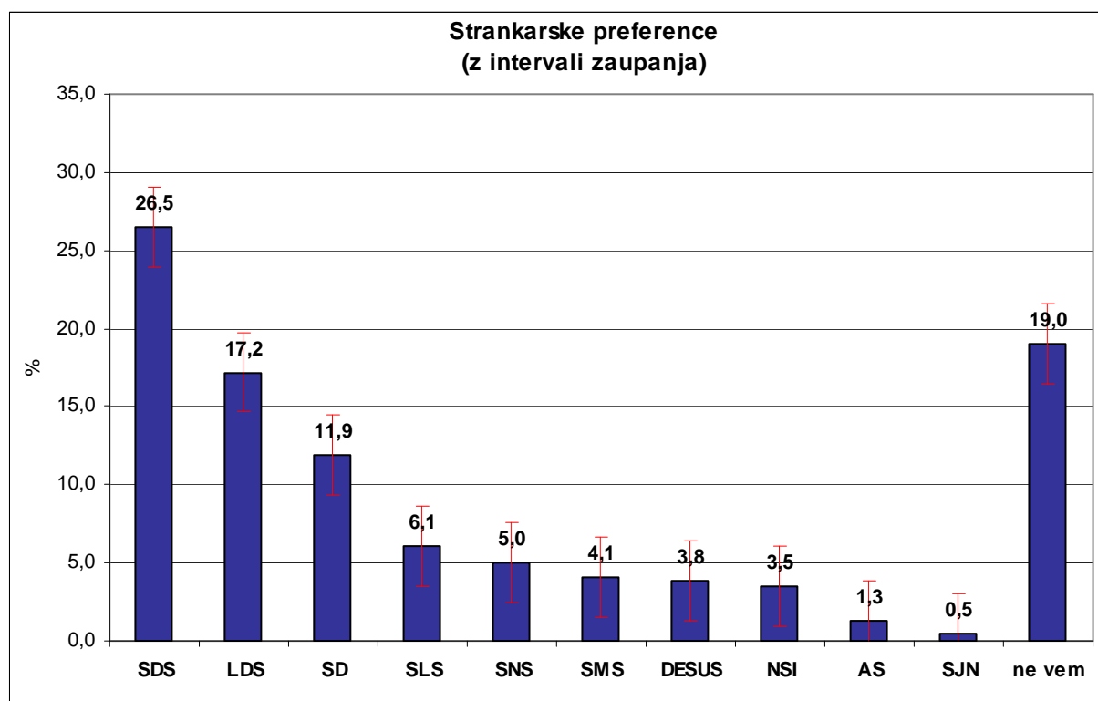
Slika 16. Strankarske preference (katero bi volil+katera vam je najbližja, prikaz v intervalu zaupanja).
