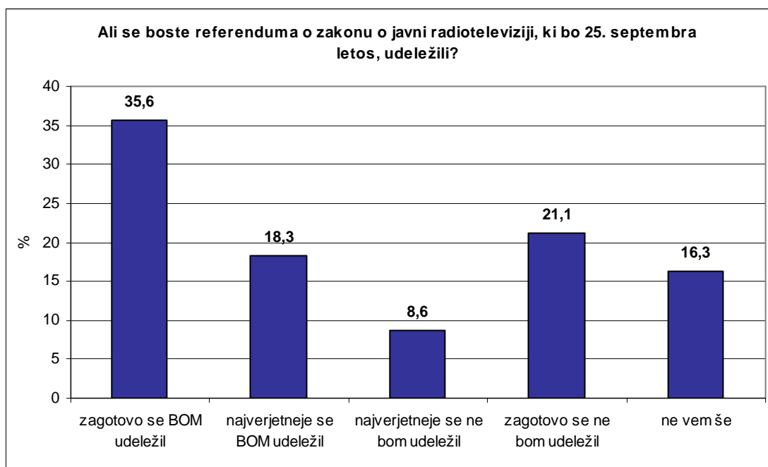
Slika 10. Udeležba na referendumu o javni RTV, 25. septembra.
