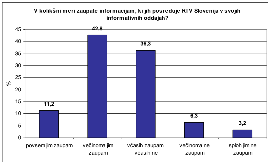
Slika 6. Zaupanje informacijam v informativnih oddajah RTV Slovenija.
