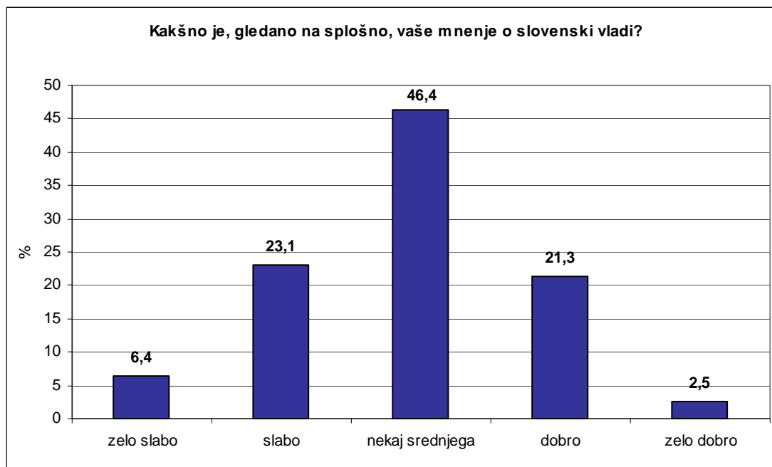
Slika 12. Splošno mnenje o slovenski vladi.
