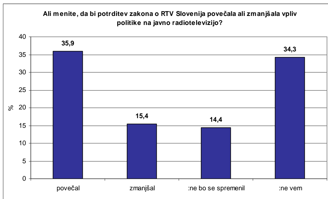
Slika 8. Mnenje o vplivu politike v primeru potrditve zakona o RTV Slovenija.
