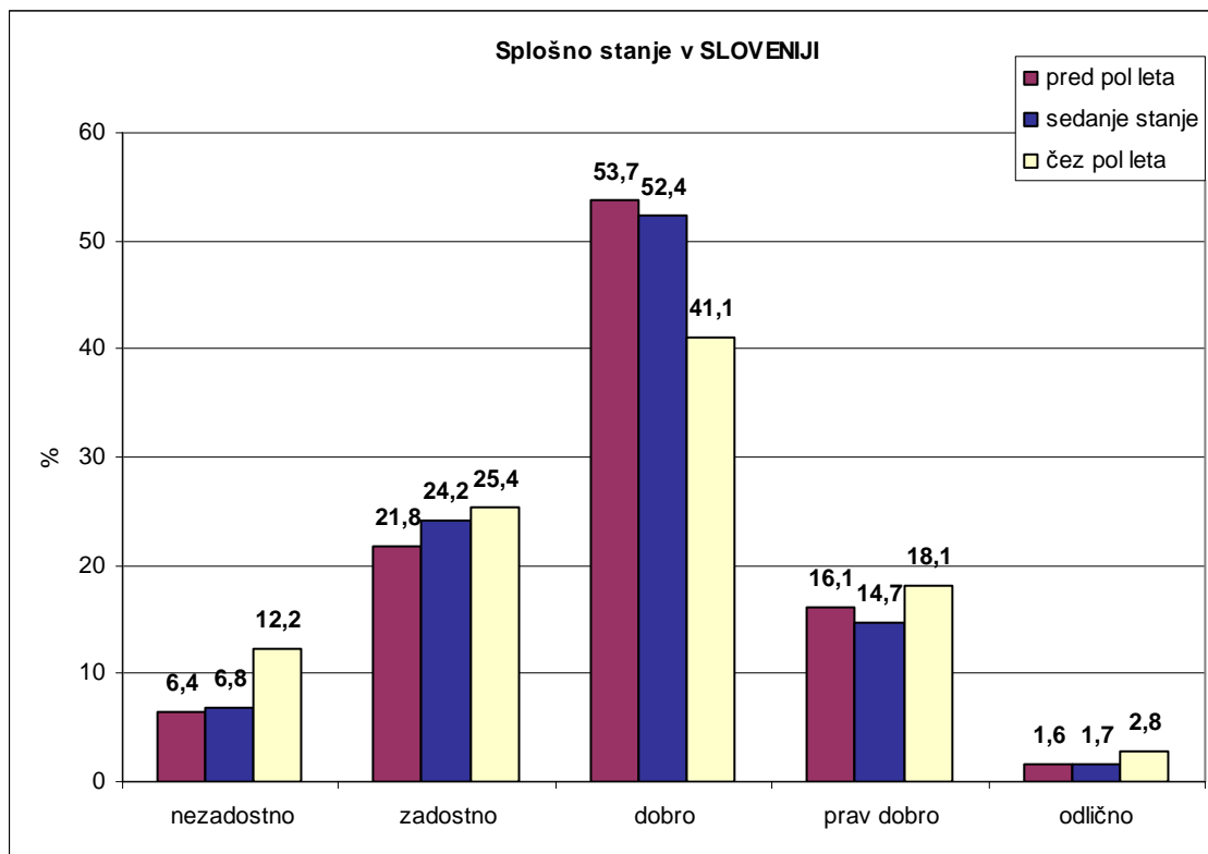
Slika 4. Ocena splošnega stanja v Sloveniji.
