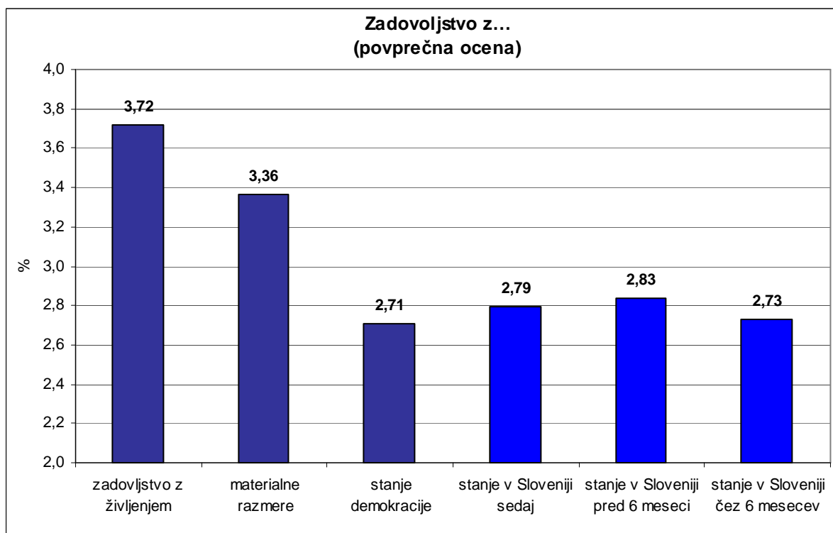
Slika 5. Povprečna ocena zadovoljstva s stanjem v Sloveniji.
