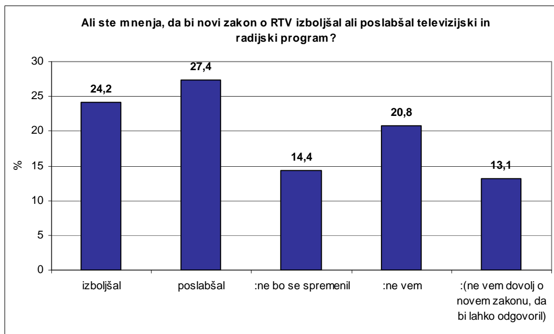
Slika 7. Mnenje o vplivu novega zakona na RTV program.
