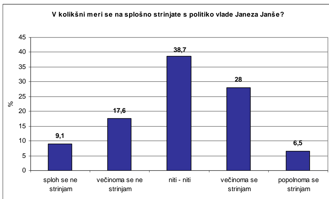
Slika 13. Strinjanje s politiko vlade Janeza Janše.
