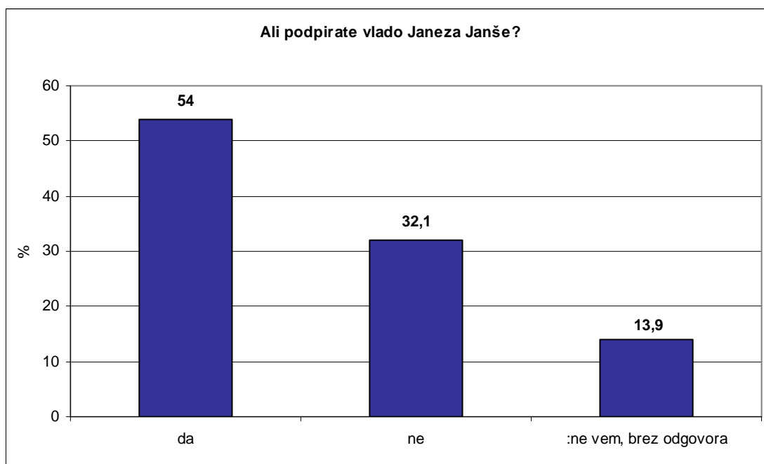
Slika 14. Podpora vladi Janeza Janše.
