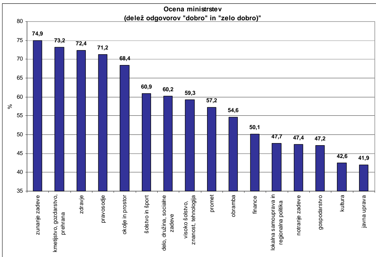
Slika 15. Ocena dela ministrstev.
