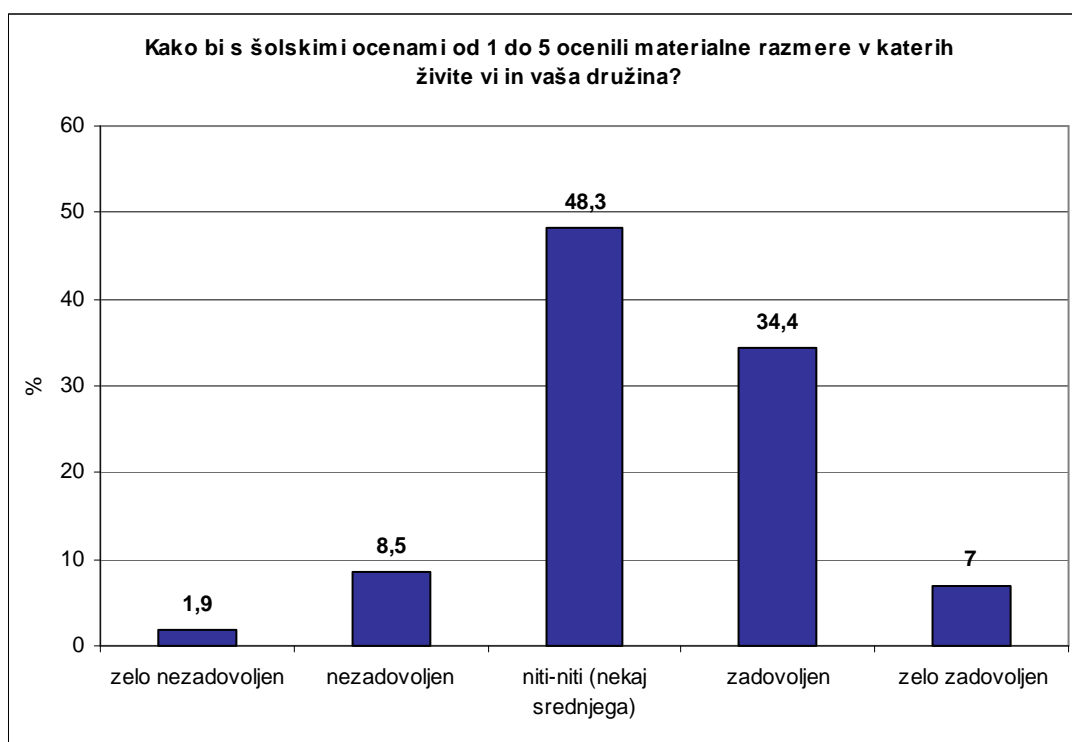
Slika 1. Zadovoljstvo z materialnimi razmerami.
